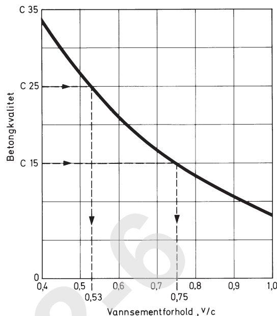
Fig. 22 Sammenheng mellom betongkvalitet og v/c-tallet for enkle betongarbeider
