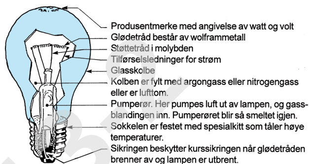
Fig. 11 a Vanlig glødelampe
