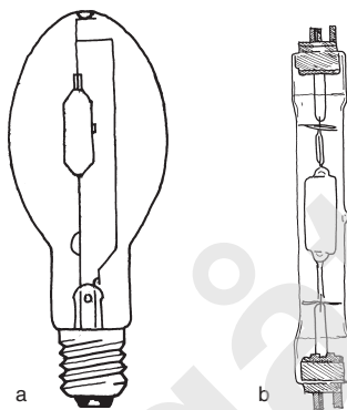
Fig. 44 a og b To typer metallhalogendampplamper a. Med skrusokkel b. Med sokkel i hver ende
