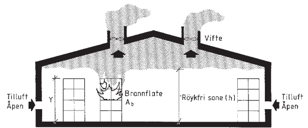
Fig. 41 Mekanisk røykventilasjon i lager
