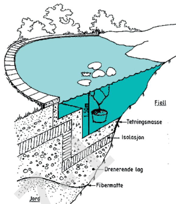
Fig. 331 b Støpt basseng
