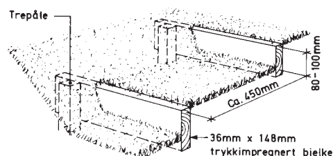
Fig. 353 Trykkimpregnerte bjelker som opptrinn.
