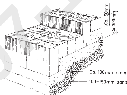
Fig. 352 b Jernbanesviller kappet på tvers.
