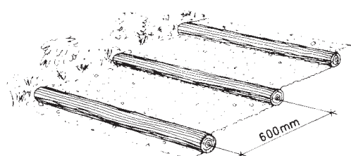
Fig. 351 Trappeveg med runde stokker og grus.
