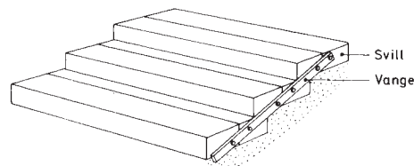
Fig. 352 a Trapp av sviller brukt på langs. Kantforsterkning er satt på langs siden.
