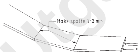
Fig. 22 a En maksimal utnyttelse av isolasjonsplatenes isolasjonsevne forutsetter god tilpassing mellom platene.
