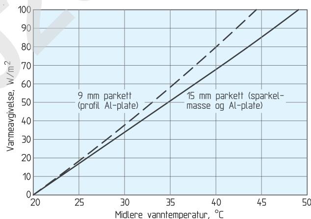
Fig. 43 a Måling av varmeavgivelse fra et lett golvvarmeanlegg med 9 og 15 mm parkett over varmerør og varmefordelingsplater. For golv med 15 mm parkett ligger varmerørene i spor i EPS-isolasjon omgitt av ledende (anhydritt) masse med heldekkende 0,5 mm Al-plate. For golv med 9 mm parkett ligger rørene i spor i porøse trefiberplater med profilerte 0,5 mm Al-plater (profilplater). Romtemperaturen er 20 °C.
