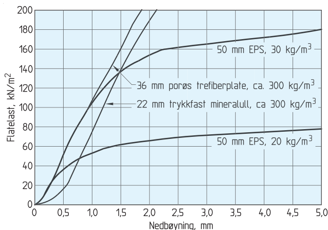
Fig. 34 b Måling av sammenheng mellom flatelast og nedbøyning for 36 mm tykk porøs trefiberplate, 20 mm trykfast mineralull og 50 mm EPS-isolasjon (20 og 30 \text{ kg/m}^3 ) Ved sammenlikning av ulike materials stivhet (ISO 844 Cellular plastics – Compression test for rigid materials – Specification) ser man bort fra initialnedbøyningen ved små laster (krum kurve).
