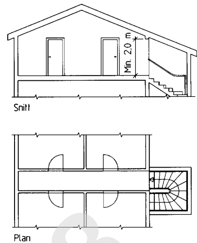
Fig. 22 b Trappeløp til påbygd areal er lagt i tilbygg utenfor hovedetasjen. Trappeløpet griper lite inn i hovedkonstruksjonene for huset og gir gode utnyttelsesmuligheter i påbygget. Løsningen krever stor høyde i påbygget.
