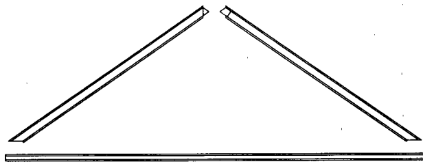
Fig. 43 a Monterbare takbind av I-bjelker
