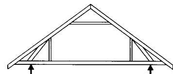
Fig 41 b A-takstol med inntreksstaver
