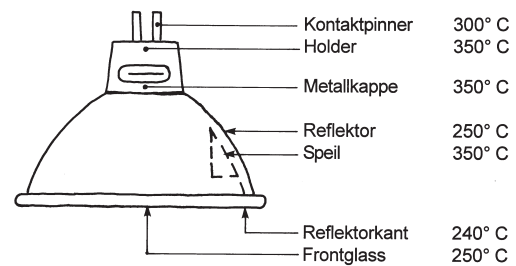
Fig. 231 a
