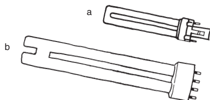
Fig. 343 a og b To typer kompaktlysør a. Topinner kompaktlysør b. Firepinners kompaktlysør
