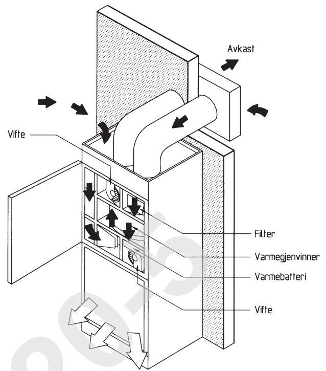
Fig. 32 Kompakte aggregater beregnet på montasje rett i yttervegg i rommene som skal ventileres Ventilasjonskapasiteten ved den hastigheten som tilfredsstiller støykravene, må være så stor at kravene til ventilasjon da er tilfredsstillt.
