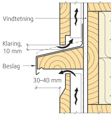
Fig. 76 Beslag for brannoppdeling av kledning
