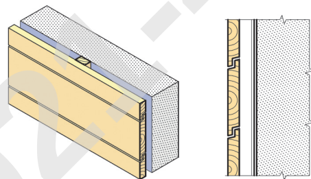
Fig. 34 Åpen, dobbeltfalset kledning
