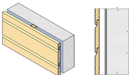
Fig. 33 Dobbeltfalset kledning med «lang» skråfals
