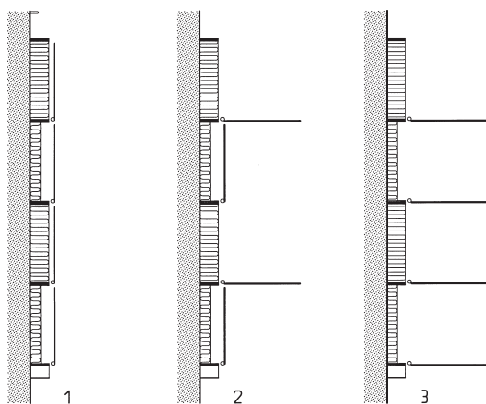
Fig. 43 b Regulerbar absorpsjon med vannrett hengslede luker på veggen [622] 1) lukkede luker – maksimal etterklangstid 2) halvparten av lukene åpne – middel etterklangstid og mange tidlige lydrefleksjoner 3) alle luker åpne – kort etterklangstid
