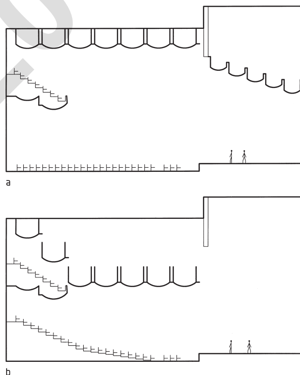
Fig. 44 a og b Sal med variabelt volum for å regulere etterklangstid a. Konsert, høyt tak, flatt golv, T = 1,6 s b. Teater, senket tak, hellende golv, ingen balkong, T = 1,3 s
