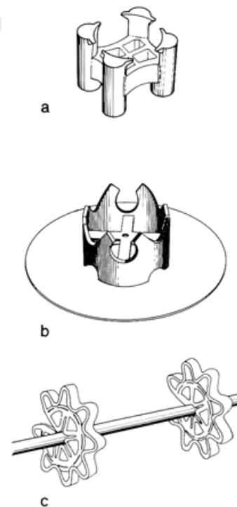
Fig. 24 a – c Armeringsstoler av plast a. Vanlig plaststol b. Plaststol med stor anleggsflate for plassering på mykt underlag c. Hjulformet armeringsstol
