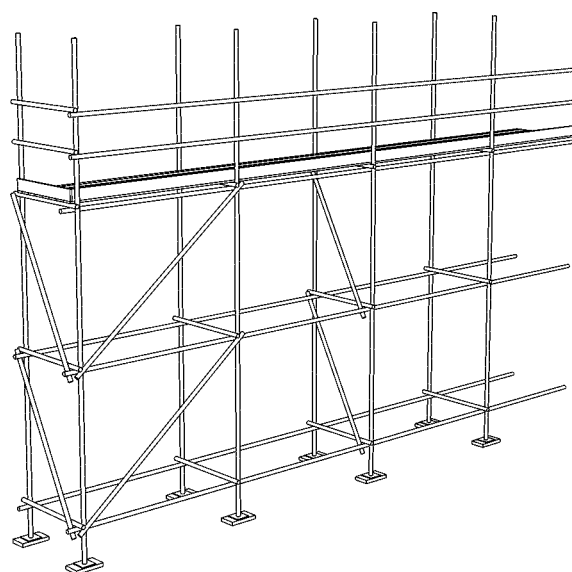
Fig. 32 Rør- og koblingsstillas
