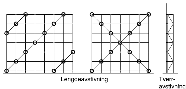
Fig. 43 Avstivning
