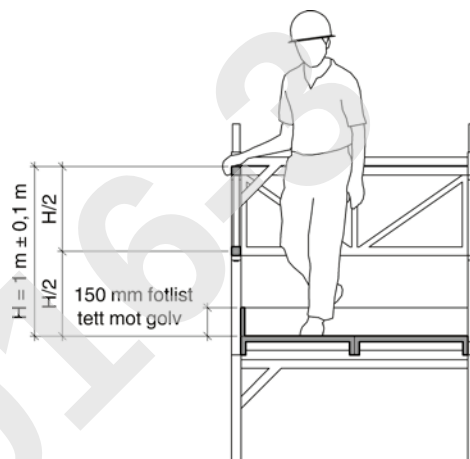
Fig. 451 Rekkverk
