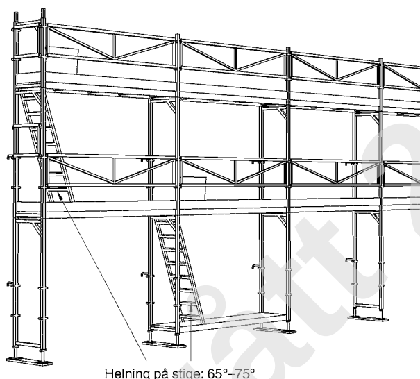
Fig. 33 Systemstillas
