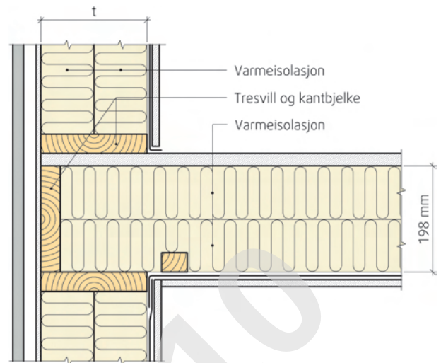
Fig. 45 a Yttervegg av bindingsverk av tre mot etasjeskiller av trebjelkelag med kuldebroverdi, \Psi , tilnærmet lik 0 for isolasjonstykkelser, t, i vegg på 98–296 mm
