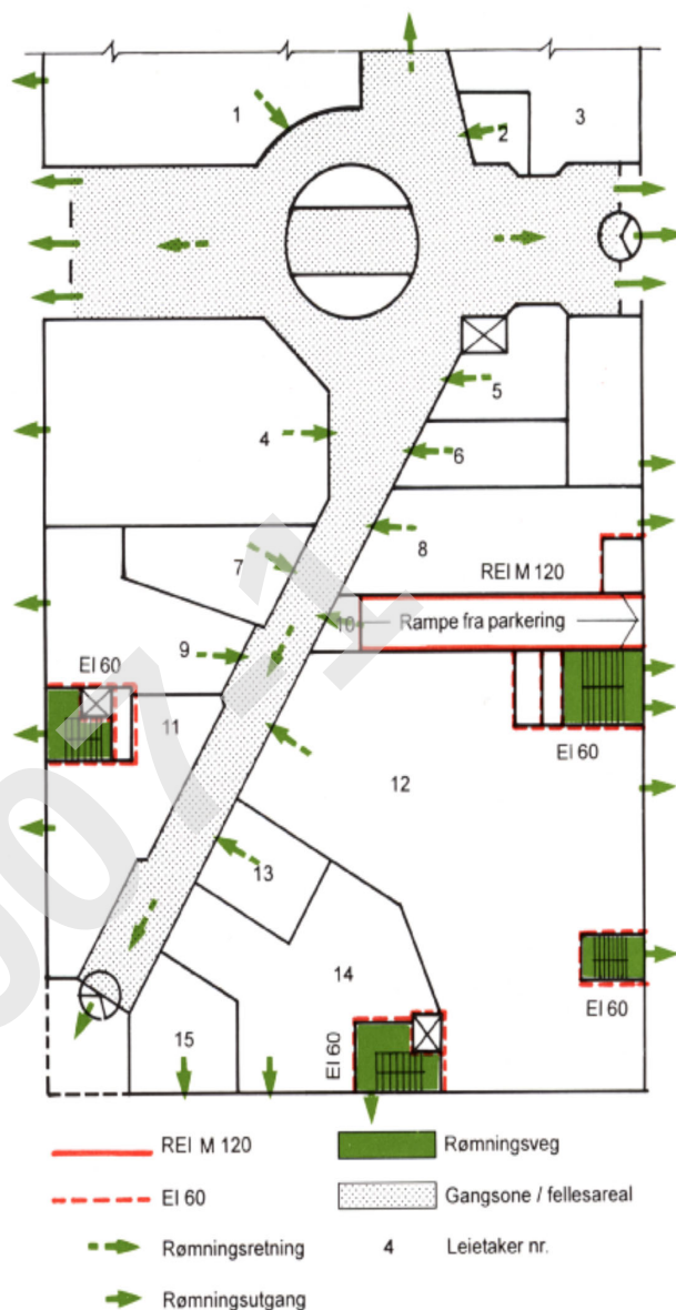
Fig. 13 a Salgslokale. Eksempel på brannteknisk tegning
