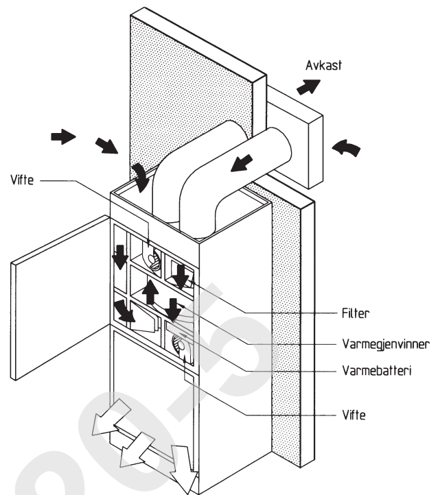
Fig. 32 Kompakte aggregater beregnet på montasje rett i yttervegg i rommene som skal ventileres Ventilasjonskapasiteten ved den hastigheten som tilfredsstiller støykravene, må være så stor at kravene til ventilasjon da er tilfredsstillt.
