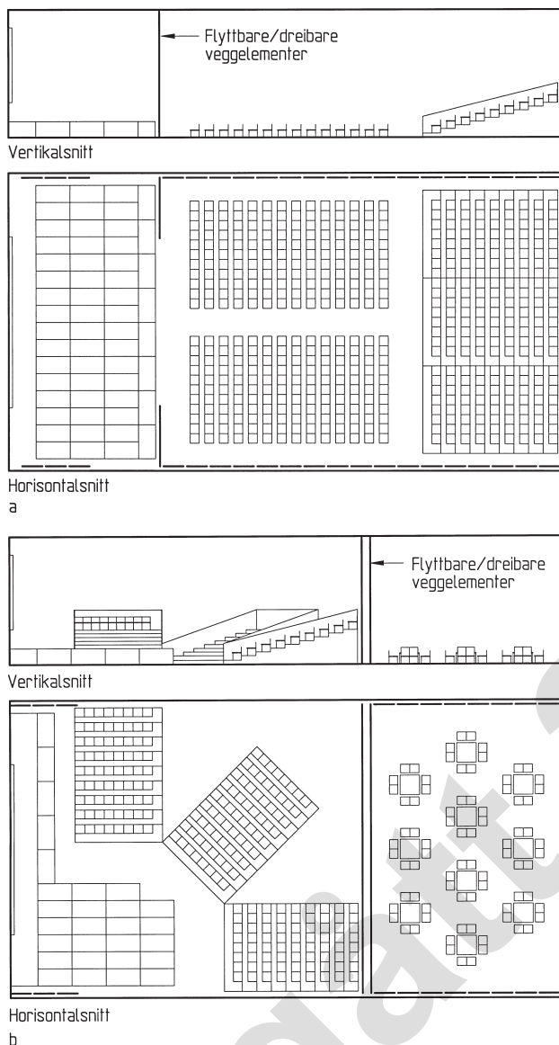
Fig. 45 a og b Sal med flyttbare og dreibare veggelementer. Salen måler 33 m x 18 m x 7,5 m a. Innredning til teater: noen veggelementer er brukt som prosce-niumramme (rammen rundt scenen) b. Veggelementene er brukt som lydisolerende dobbeltvegg. Sam-tidige funksjoner her er eksperimentalteater og bridgeturning.
